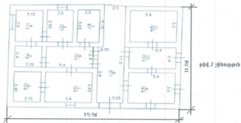
2 Շինությունների սխեմատիկ հատակագծերը (չափերը մ-ով)
